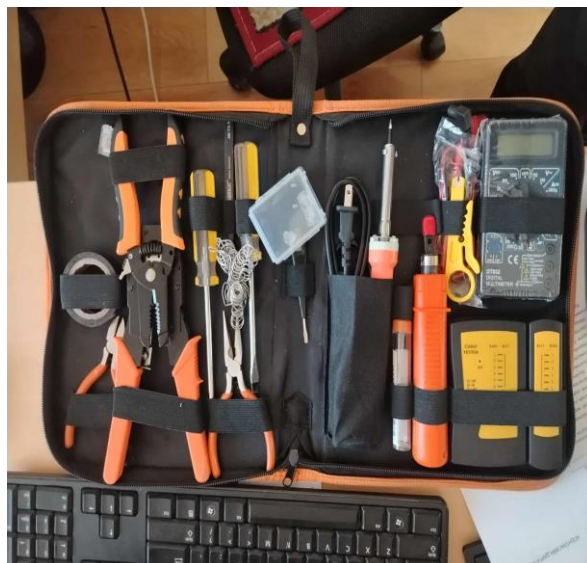
сүлжээ болон засварын тоног
